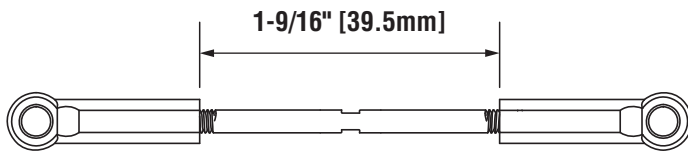
TIE ROD
