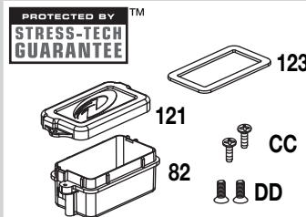
Radio Box Set DTXC8393
